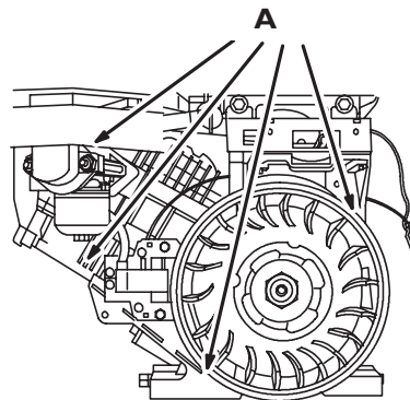
Figura 15 — Sistema de Refrigeración de Aire A - Limpie estas Areas
