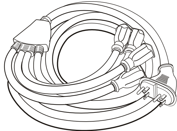
Figura 6 — Juego de Cables del Adaptador del Generador
